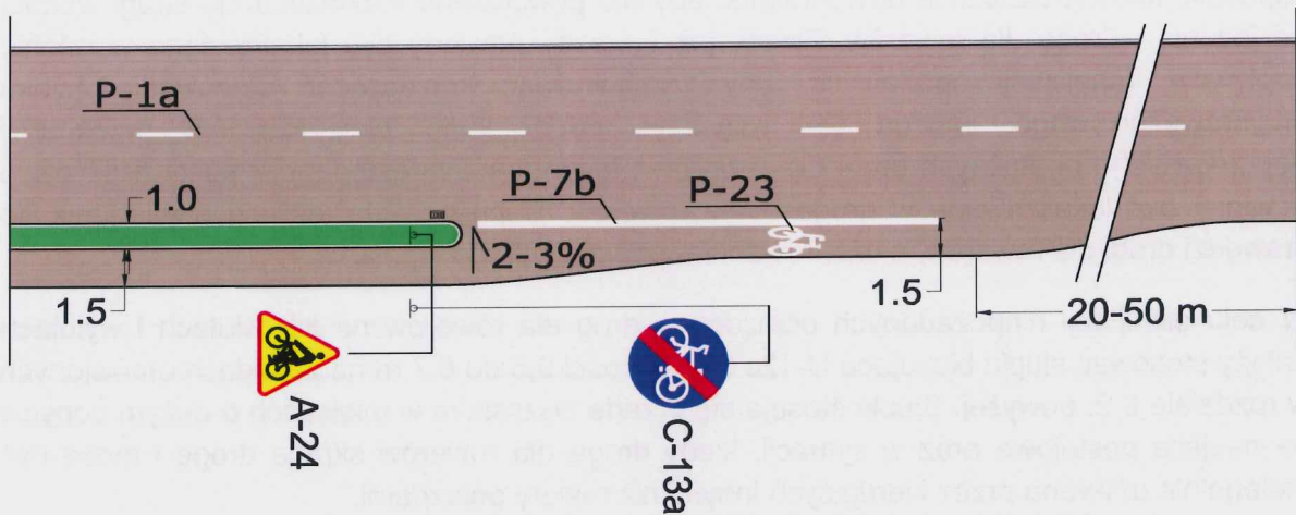
Rys. 14. Koniec jednokierunkowej drogi dla rowerów
