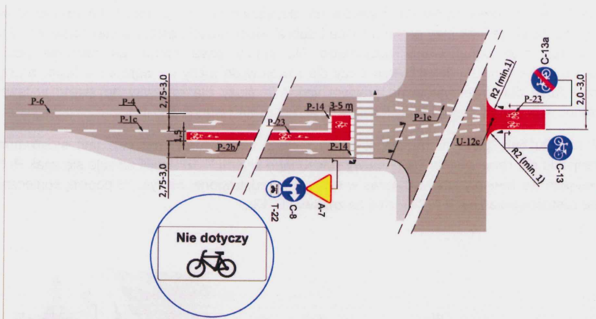
Rys. 18A. Lokalizacja pasów ruchu dla rowerów na wlocie skrzyżowania. Widoczna śluza klasyczna do jazdy na wprost i w lewo. Zamiast przejazdów dla rowerzystów (znak P-11) zastosowano oznakowanie poziome w postaci linii P-1e. W konsekwencji znak A-7 na wlocie drogi dla rowerów staje się zbędny.
