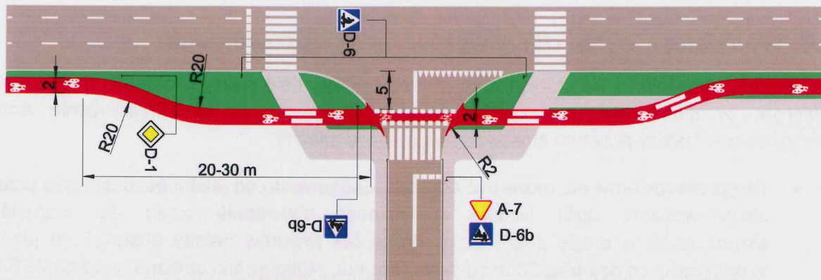
Rys. 19. Poprawny przebieg drogi dla rowerów w rejonie skrzyżowania: duże promienie łuków w dużej odległości od przejazdu dla rowerzystów. Zwracają uwagę wyokrąglenia na styku drogi dla rowerów i jezdni ogólnodostępnej.
