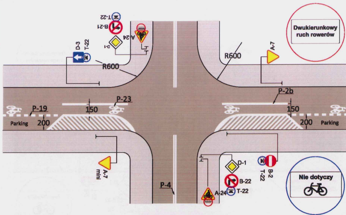
Rys. 3. Przykładowa organizacja dwukierunkowego ruchu rowerowego w jezdni jednokierunkowej – skrzyżowanie z ustalonym pierwszeństwem.
