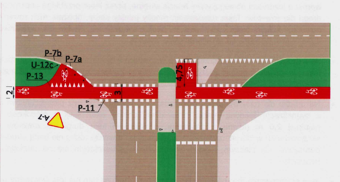
Rys. 20. Droga dla rowerów i przejazdy dla rowerzystów ze śluzami do skrętu w stronę skrzyżowania (pośrodku) i do skrętu na drodze dla rowerów (w lewym narożniku) umożliwiającymi bezpieczne pokonanie skrzyżowania na relacjach nie obsługiwanych drogami dla rowerów. Część oznakowania pionowego pominięto.
