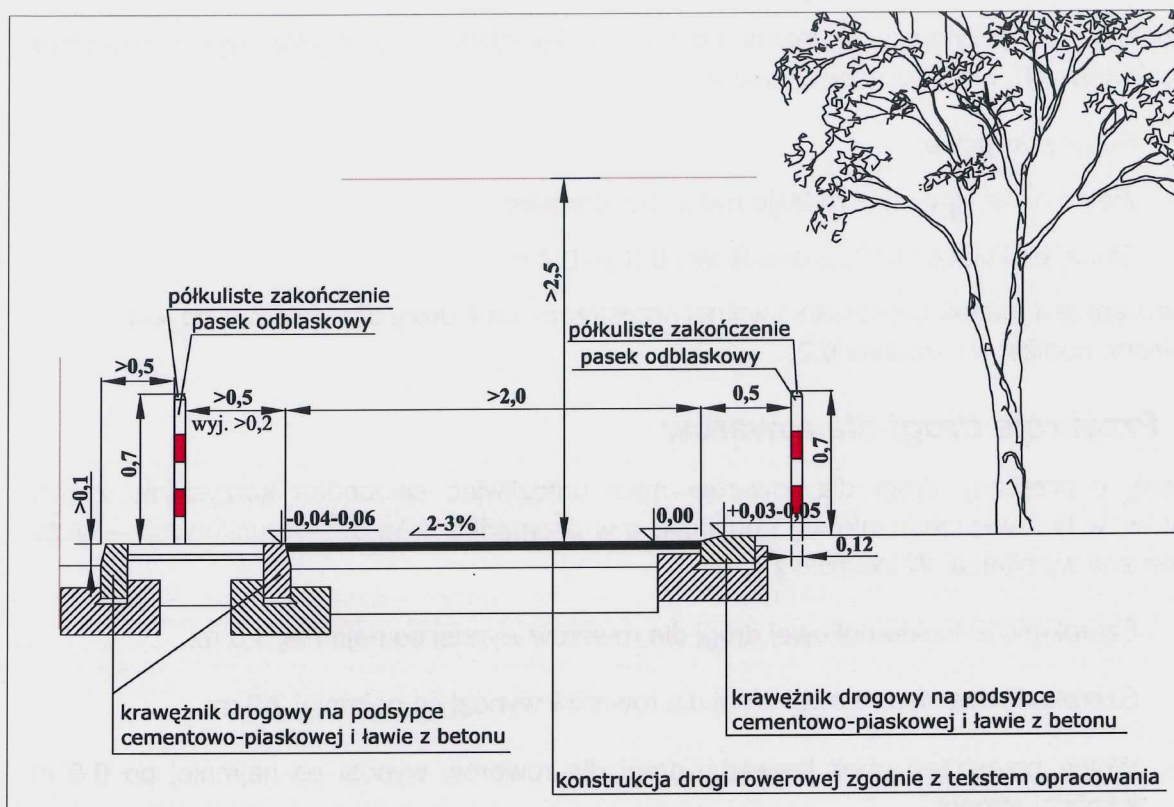
Rys. 7C. Kolejny przykład rozwiązania konstrukcyjnego drogi dla rowerów - przekrój poprzeczny dwukierunkowej drogi dla rowerów o nawierzchni bitumicznej, wariant zamknięty z obu stron krawężnikami drogowymi, w tym leżącym krawężnikiem oddzielającym ją od przylegającego chodnika.
