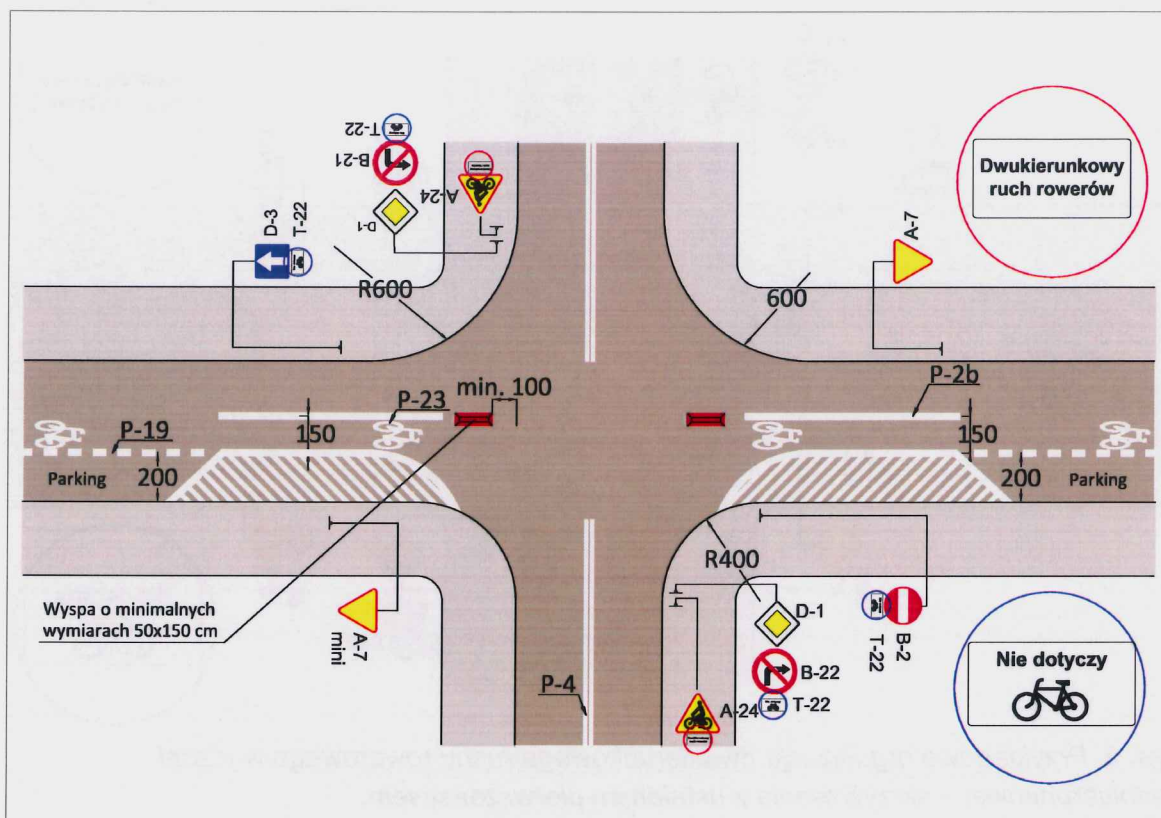
Rys. 4. Jeśli w związku z dużym natężeniem ruchu samochodowego na relacji skrzyżnej zachodzi ryzyko zajeżdżania rowerzystom drogi, można na wlocie umieścić wyspę dzielącą (także ze słupkiem U-5b, patrz rys. 6).
