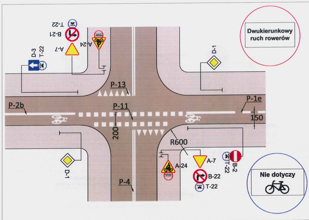
Rys. 5. Kontrapas wyznaczony w jezdni jednokierunkowej na skrzyżowaniu z ustalonym pierwszeństwem. Jeśli na skrzyżowaniu występuje duże natężenie pojazdów samochodowych na relacji skrętnej z drogi z pierwszeństwem, na wlocie umieszcza się wyspę dzielącą ze słupkiem U-5b (patrz rys. 4 i rys. 6). Zamiast przejazdu dla rowerzystów (linia P-11) można zastosować oznakowanie poziome jak na rys. 3A (linia P-1e).
